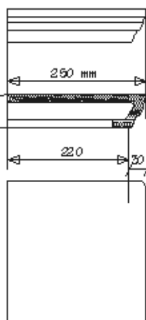
SEDACIA ROHOVÁ HRANATÁ 1123
