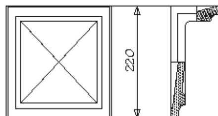
OBKLADOVÁ ROHOVÁ "L" 1278
